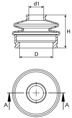
KESİT A-A
